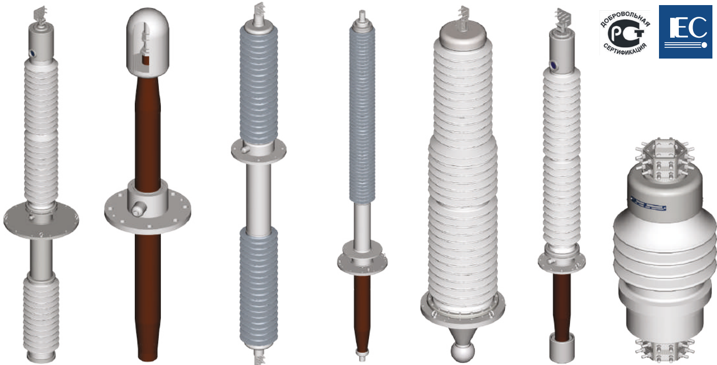
断路器套管（油-气） 电压：35-220千伏 电流：1000-3150安
